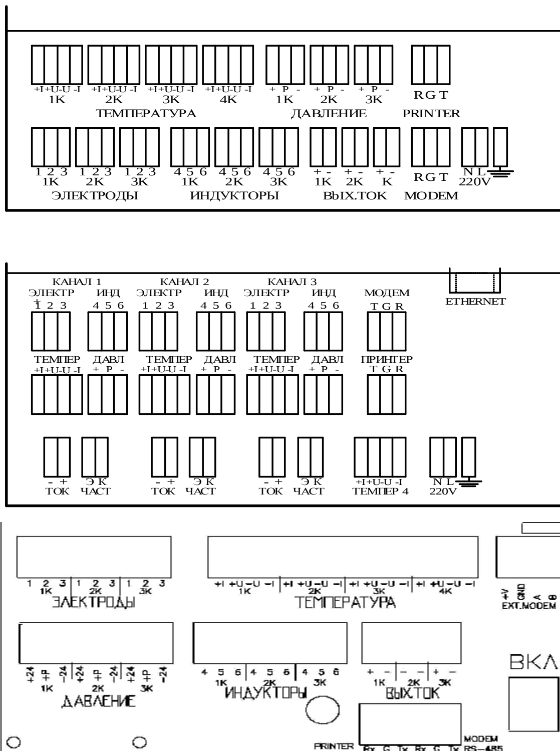
Рис.1 Блок электронный на 1 – 3 канала (варианты)
