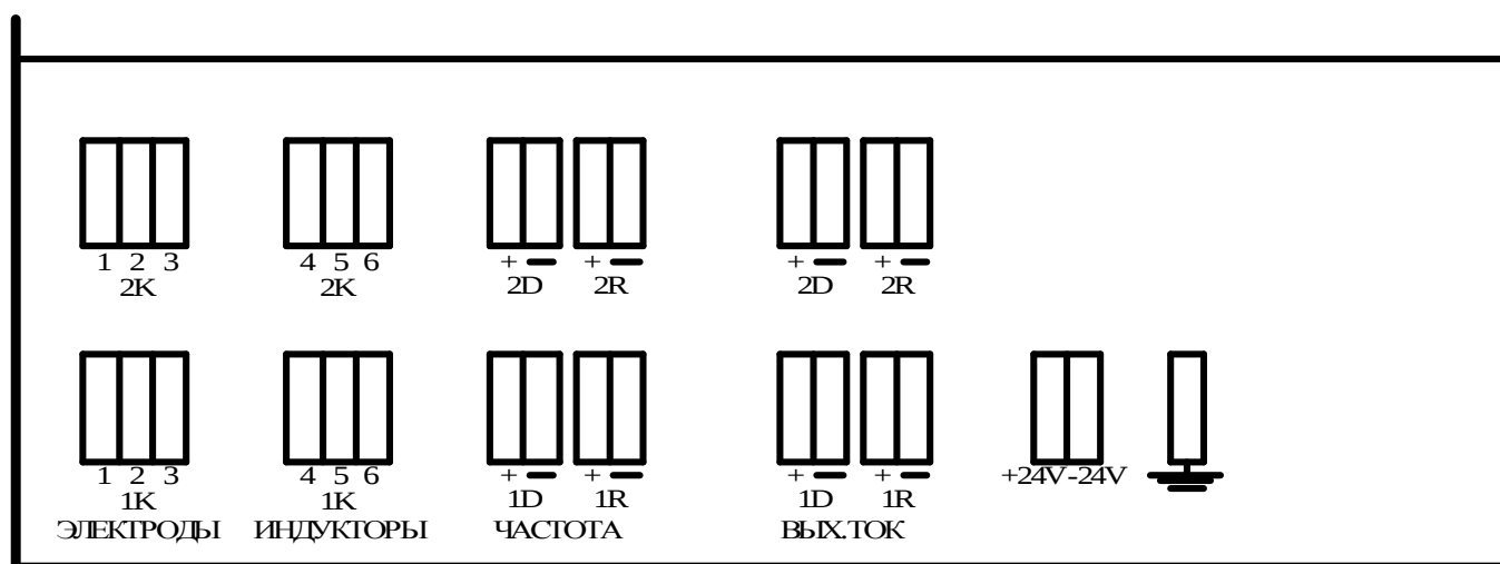
Рис.4 Блок ПНЧ
