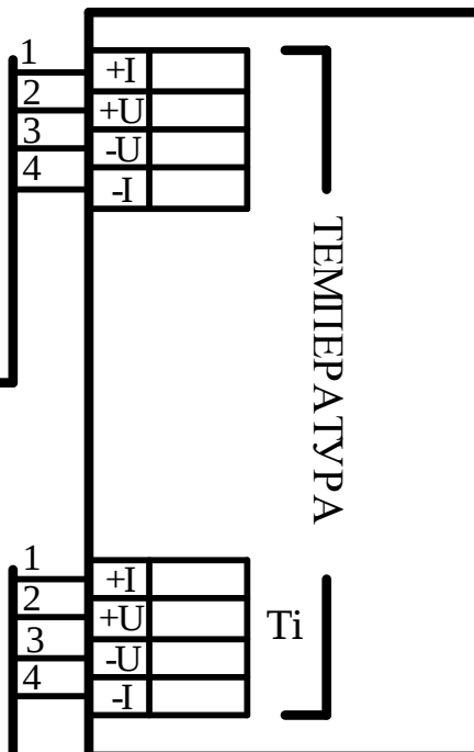
Блок электронный
